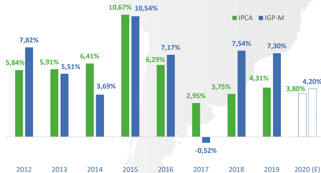
Inflação
