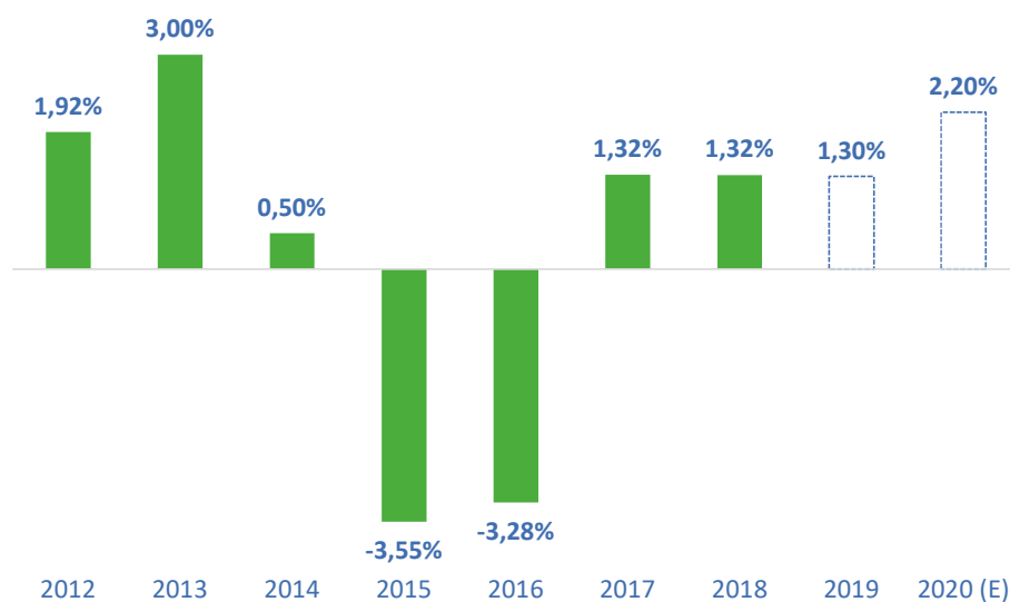
PIB
