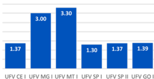
Figura 9 - Capacidade Instalada por UFV (MWp)
